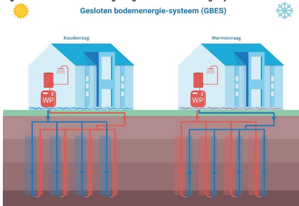
Figuur 1: Schematische weergave gesloten bodemenergiesysteem
