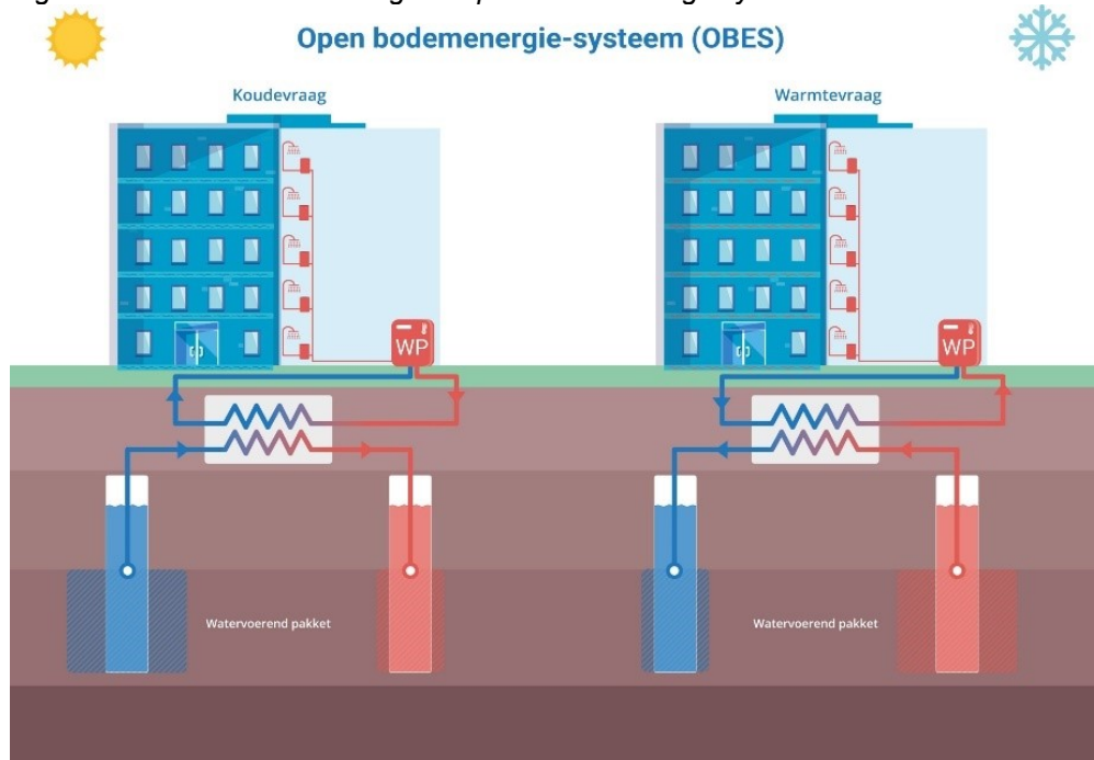
Figuur 2: Schematische weergave open bodemenergiesysteem
